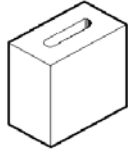
10-03 190 x 190 x 90 Half block 4.1kg 260 per pallet
